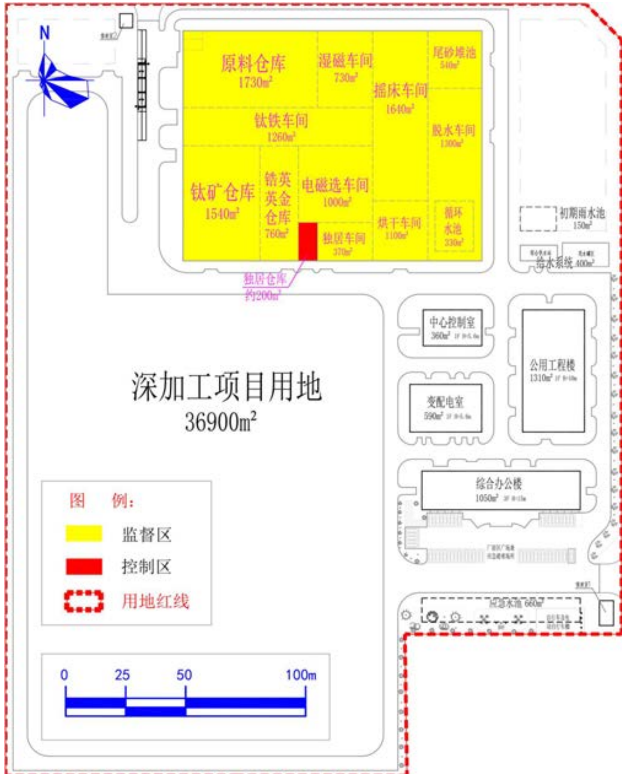
图 6.8-1 厂区辐射分区管理布局图
