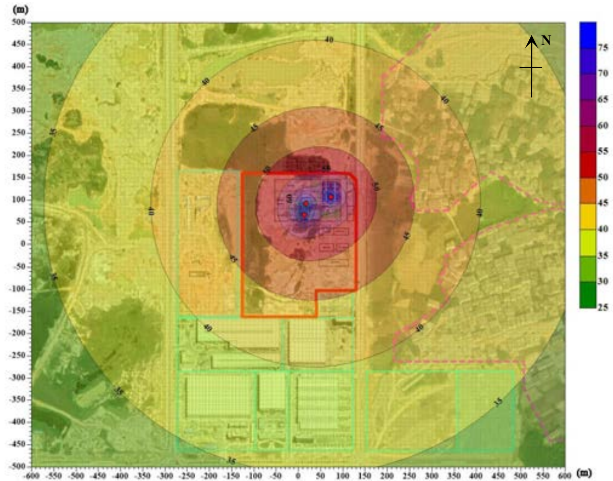
图 5.5-2 主要声源贡献值等声级线图（处理前）（单位：dB(A)）
