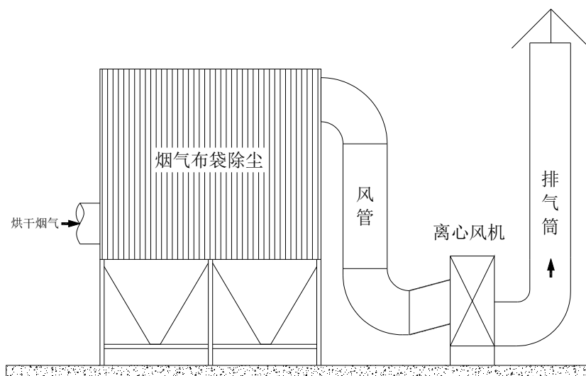
图 6.4-3 干选车间布袋除尘系统示意图
