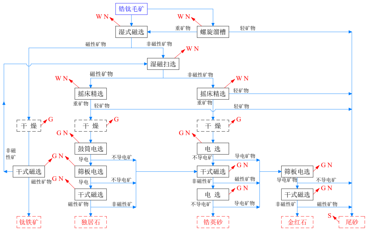
图 3.6-1 新建项目选矿工艺主要产污环节图
