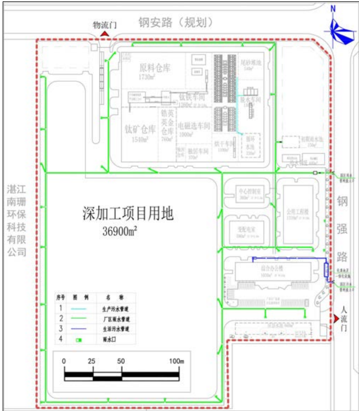
图6.2-4 厂区雨水、污水管道示意图
