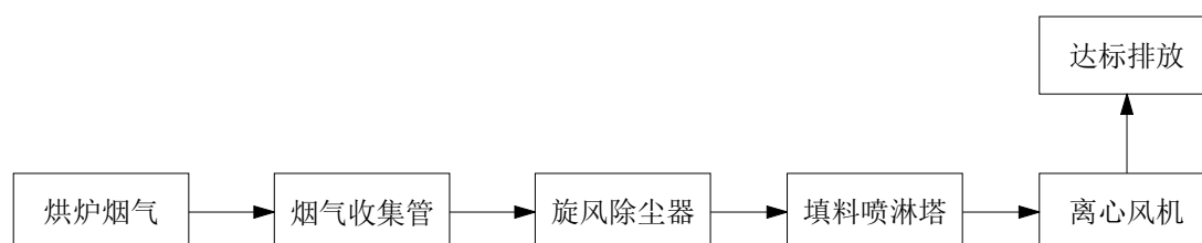
图7.4-1 “旋风+湿法除尘”工艺流程图
