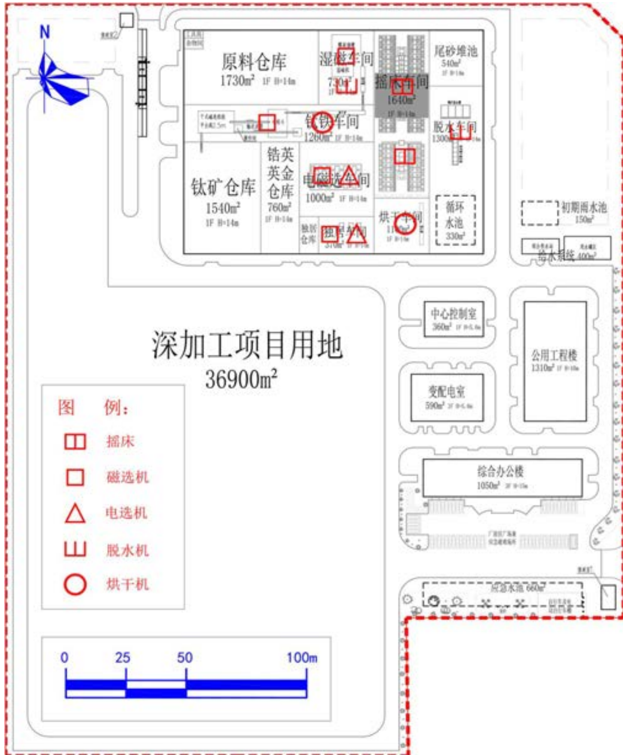
图 3.7-1 项目主要声源位置分布示意图
