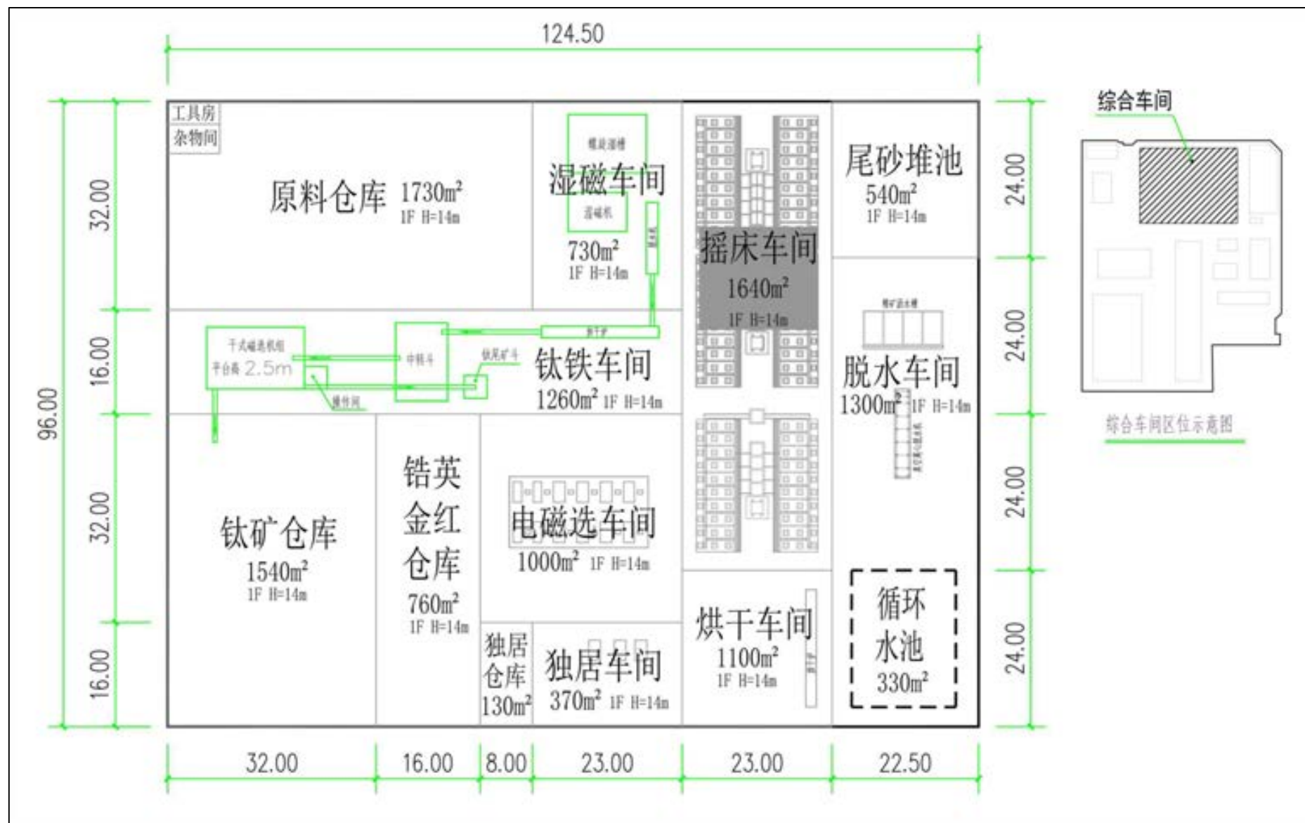
图 3.4-2 综合车间选矿及配套设施平面布置图
