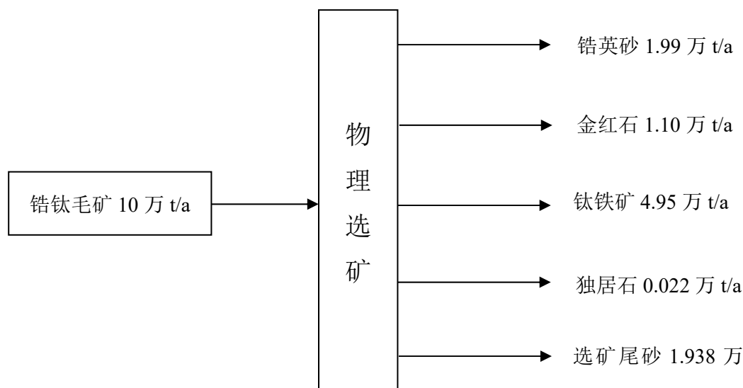
图 3.5-2 选矿工艺过程物料平衡图
