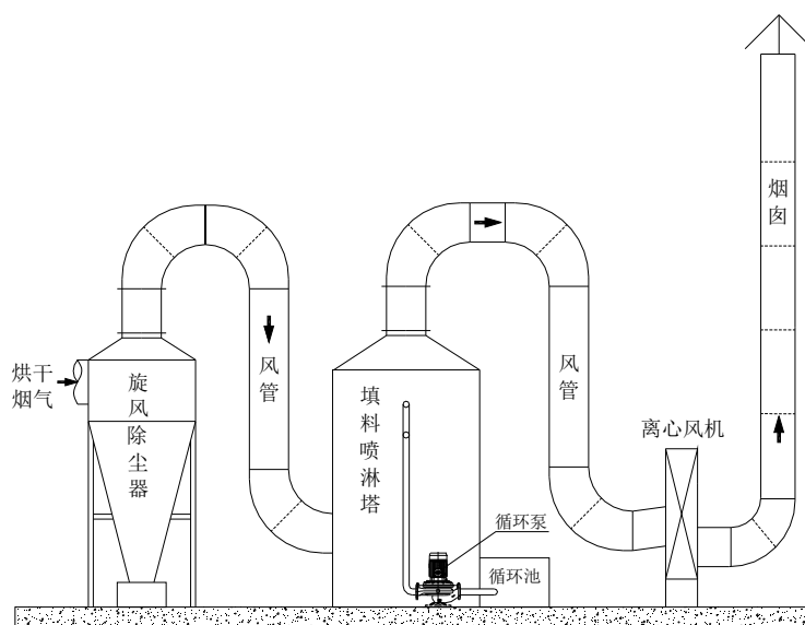
图 6.4-2 “旋风除尘+湿法除尘”系统组成图
