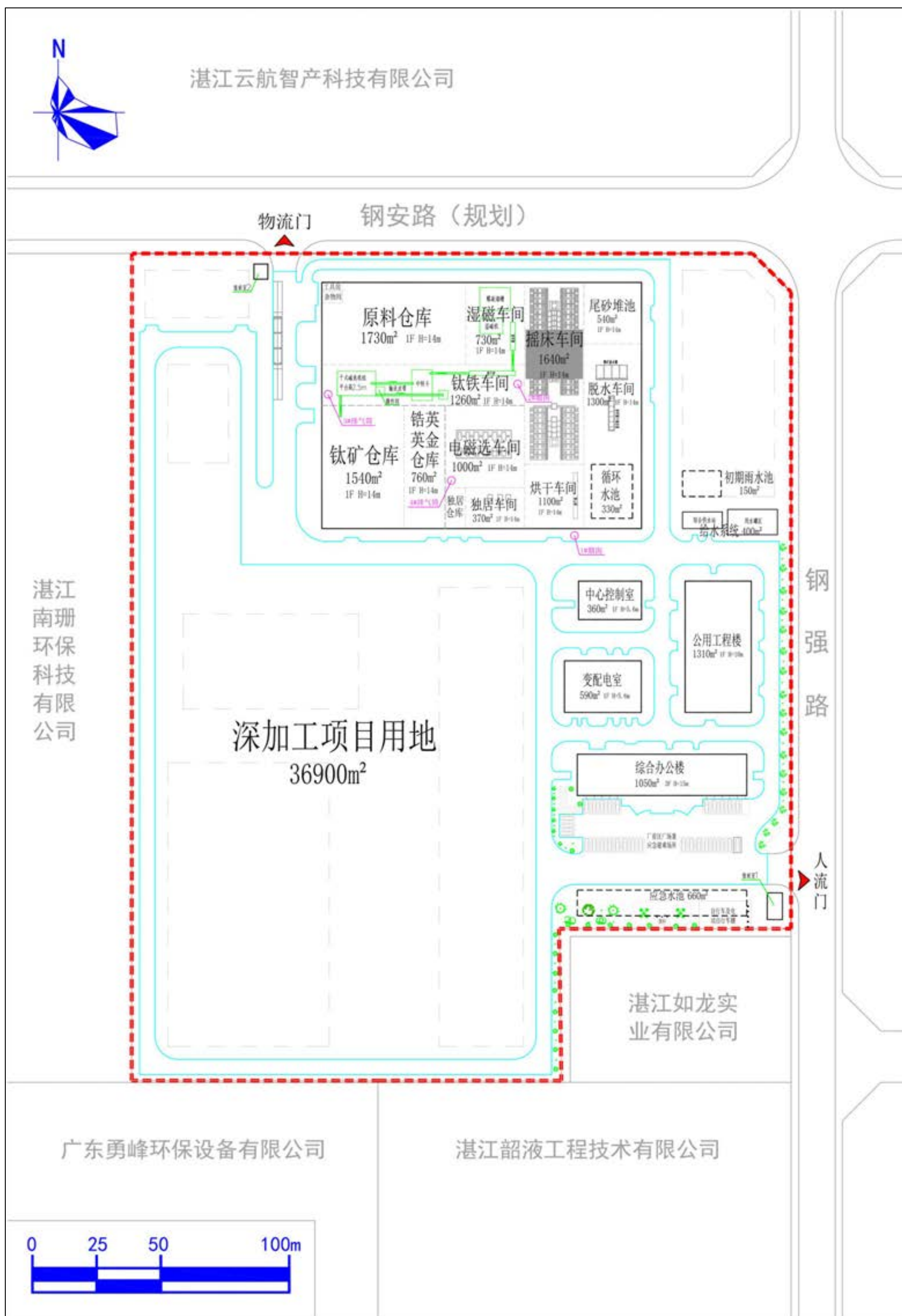
图 3.4-1 本项目总平面布置图
